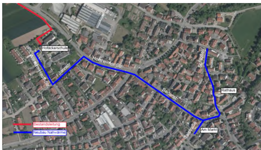
Abbildung: Trassenverlauf Nahwärme Sersheim
